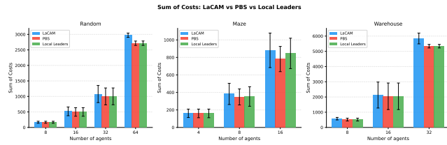
Slika 2: Vsota stroškov (SoC): LaCAM, PBS in Local Leaders na naključnih, labirintnih in skladiščnih zemljevidih. Napake kažejo standardno deviacijo čez 3 semena.
