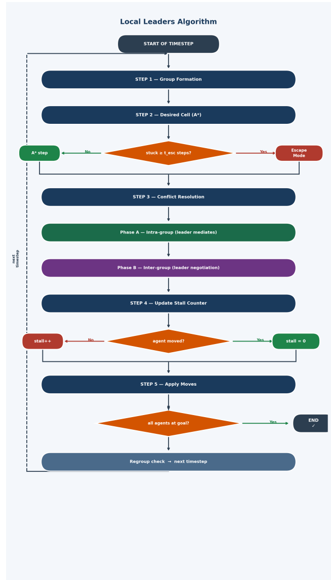
Slika 1: Diagram poteka algoritma Local Leaders: dinamično oblikovanje skupin, določitev vodje, A^* načrtovanje in dvofazna razrešitev konfliktov (znotraj skupinska posredovanost vodje, nato medskupinsko pogajanje vodij).
