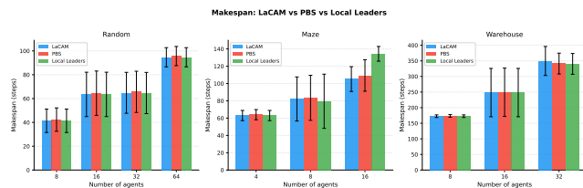
Slika 3: Makespan: LaCAM, PBS in Local Leaders. Na naključnih in skladiščnih zemljevidih so vsi trije algoritmi praktično identični; na labirintnih PBS doseže makespan 109 pri 16 agentih (vs. LaCAM 105), Local Leaders pa 134, kar je posledica delno neuspešnih instanc.
