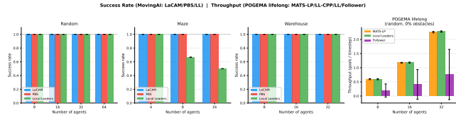
Slika 5: Levo: stopnja uspeha LaCAM, PBS in Local Leaders na MovingAI enkratnih (ang. one-shot ) scenarijih. Desno: pretočnost v neprekinjenih (ang. lifelong ) scenarijih MATS-LP, Local Leaders in Follower na POGEMA (naključni zemljevidi, 0 % ovir).
