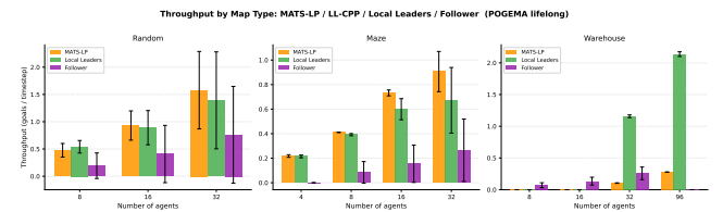
Slika 8: Pretočnost v neprekinjenih (ang. lifelong ) scenarijih MATS-LP, Local Leaders in Follower po tipu zemljevida (naključni, labirint, skladišče). Na skladiščnih zemljevidih Local Leaders dosega do 10× višjo pretočnost kot MATS-LP.
