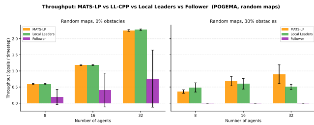
Slika 6: Pretočnost v neprekinjenih (ang. lifelong ) scenarijih MATS-LP, Local Leaders in Follower na naključnih zemljevidih pri 0 % (levo) in 30 % (desno) gostoti ovir. Rezultati Local Leaders so iz C++ implementacije. Pri 30 % ovirah Local Leaders ostaja konkurenčen pri manjšem številu agentov, a zaostaja pri 32 agentih.
