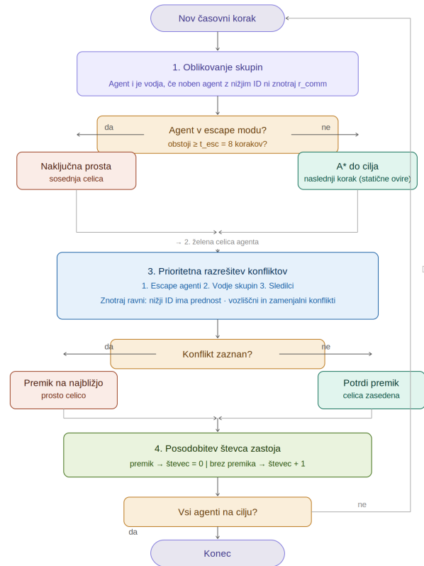
Slika 1: Diagram poteka algoritma Local Leaders: dinamično oblikovanje skupin, določitev vodje, A* načrtovanje in prioritna razrešitev konfliktov.
