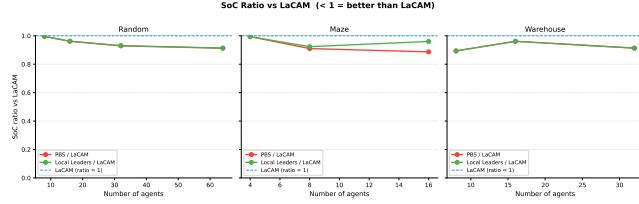
Slika 7: Razmerje SoC (Local Leaders / LaCAM) po tipu zemljevida. Vrednost pod 1 pomeni, da Local Leaders doseže nižji SoC kot LaCAM.
