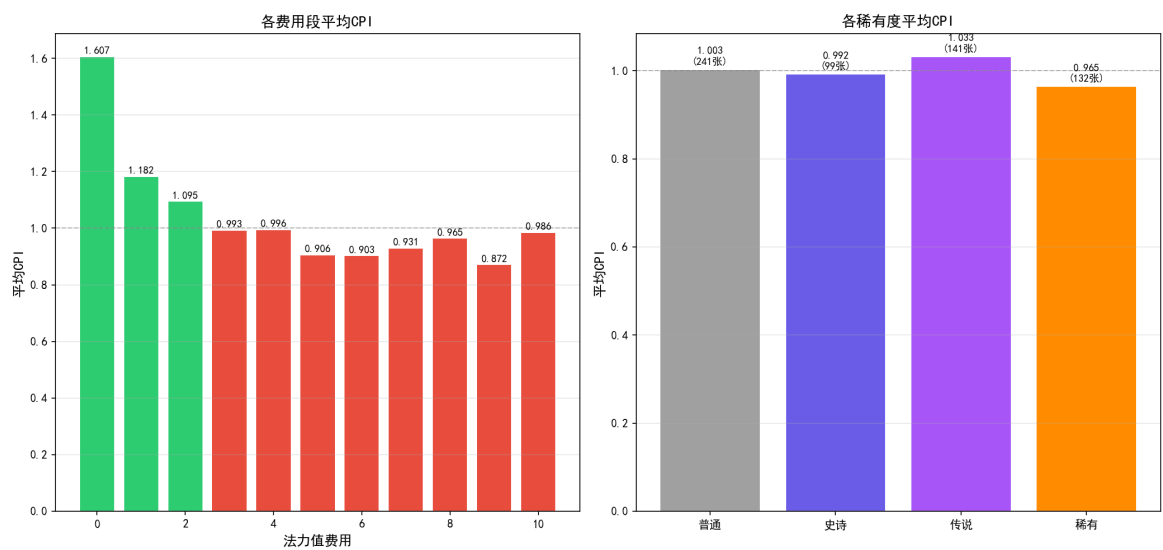
图3：CPI按费用段和稀有度的分布
