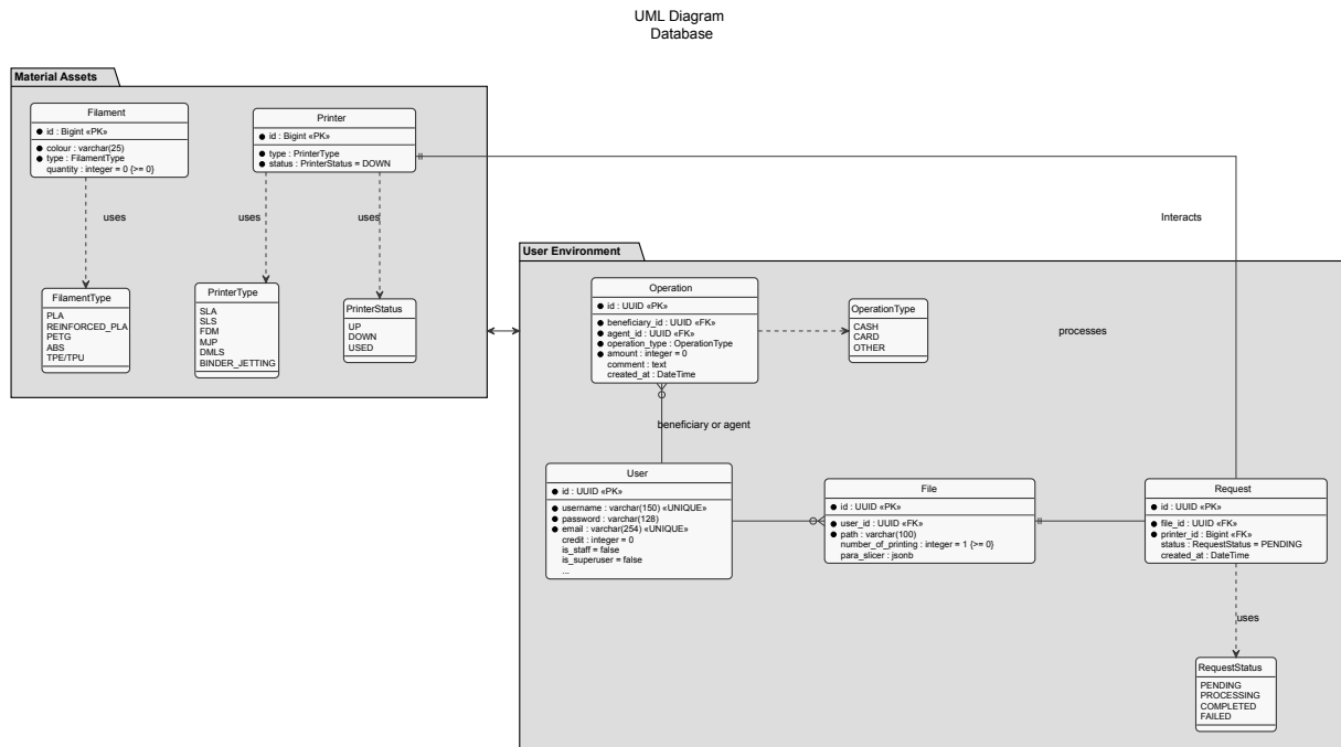
Figure 1: Schema de base de données
