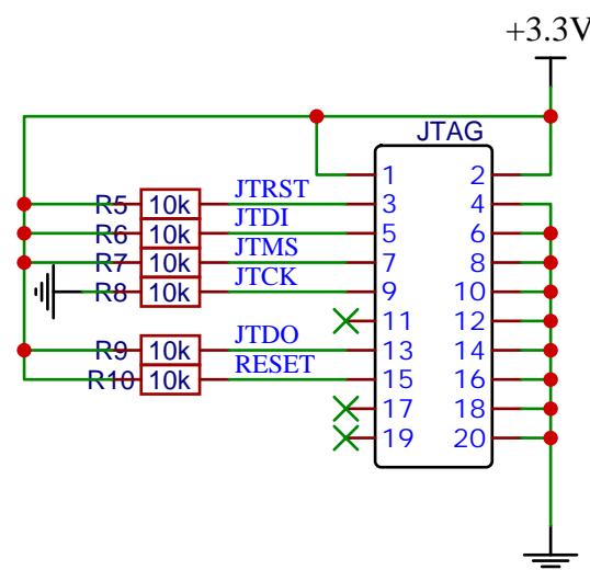
JTAG/SWD调试接口电路
