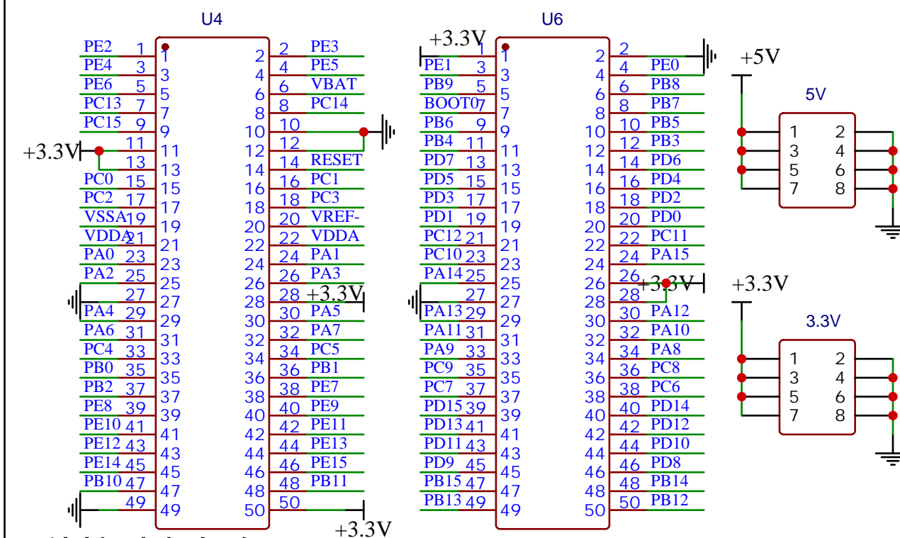
外扩引脚电路
