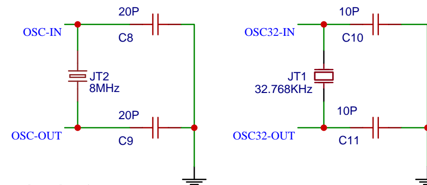
晶振电路
