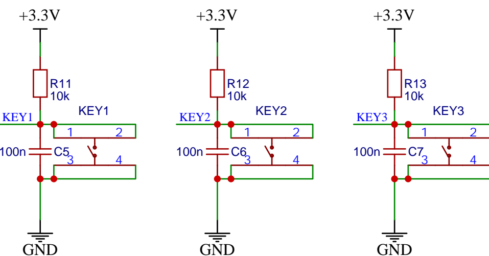
按键电路
