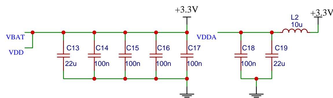
电源电路
