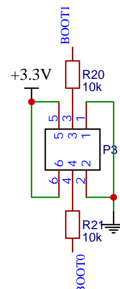
主控电路
