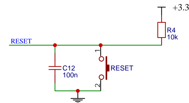
复位电路
