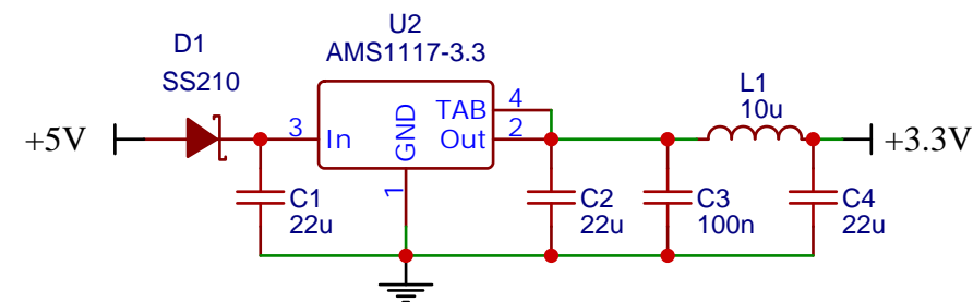
稳压电路
