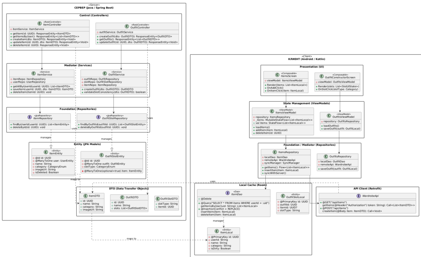
Рисунок 7. Детальная диаграмма классов проектирования
