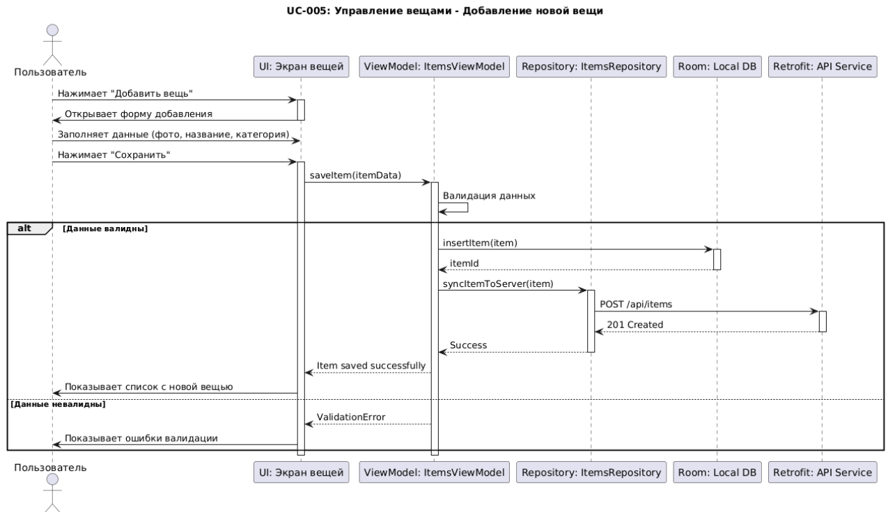
Рисунок 6. Пример диаграммы последовательности для UC-005
