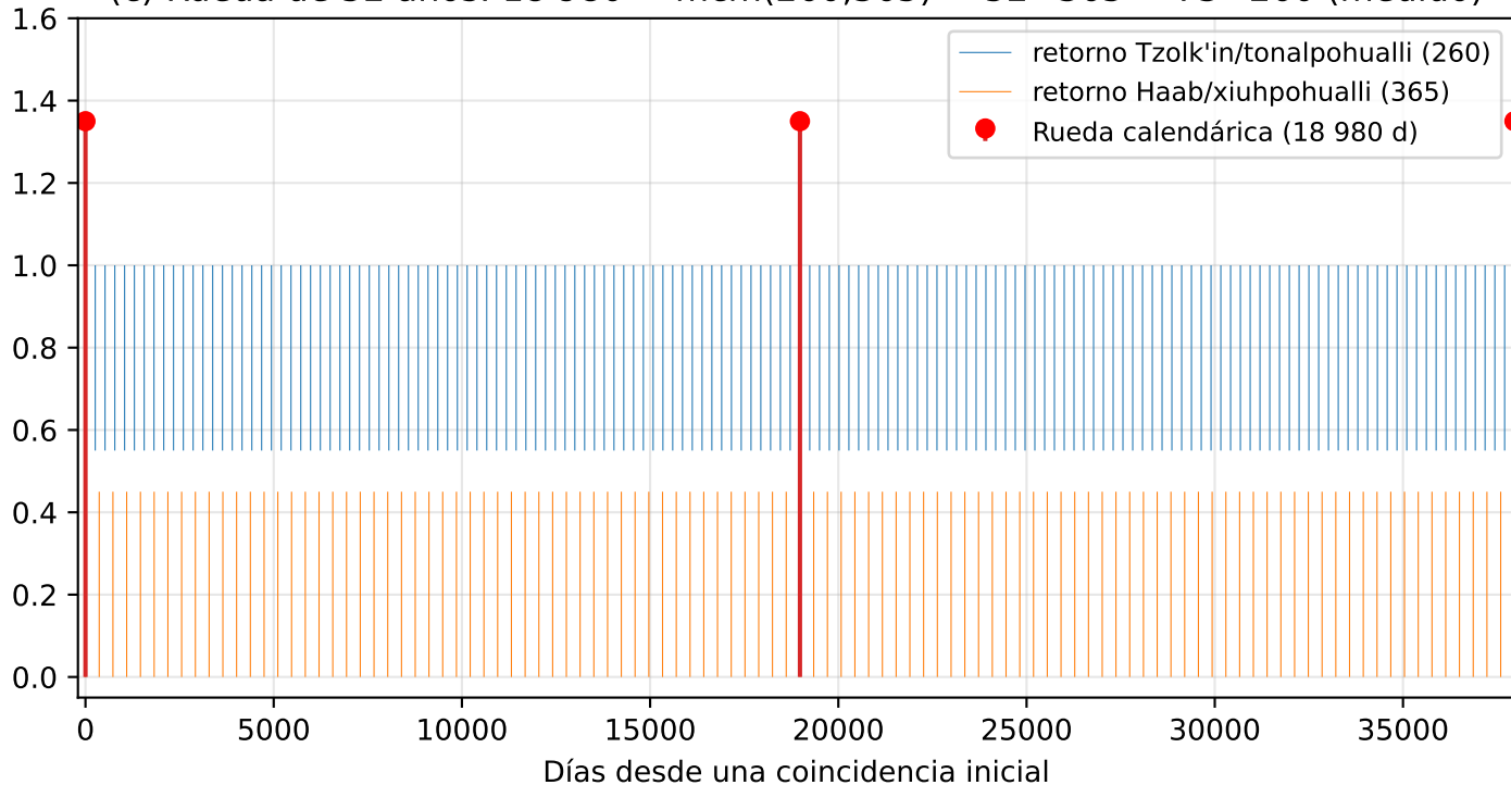
(c) Rueda de 52 años: 18\,980 = \text{mcm}(260, 365) = 52 \times 365 = 73 \times 260 (medido)
