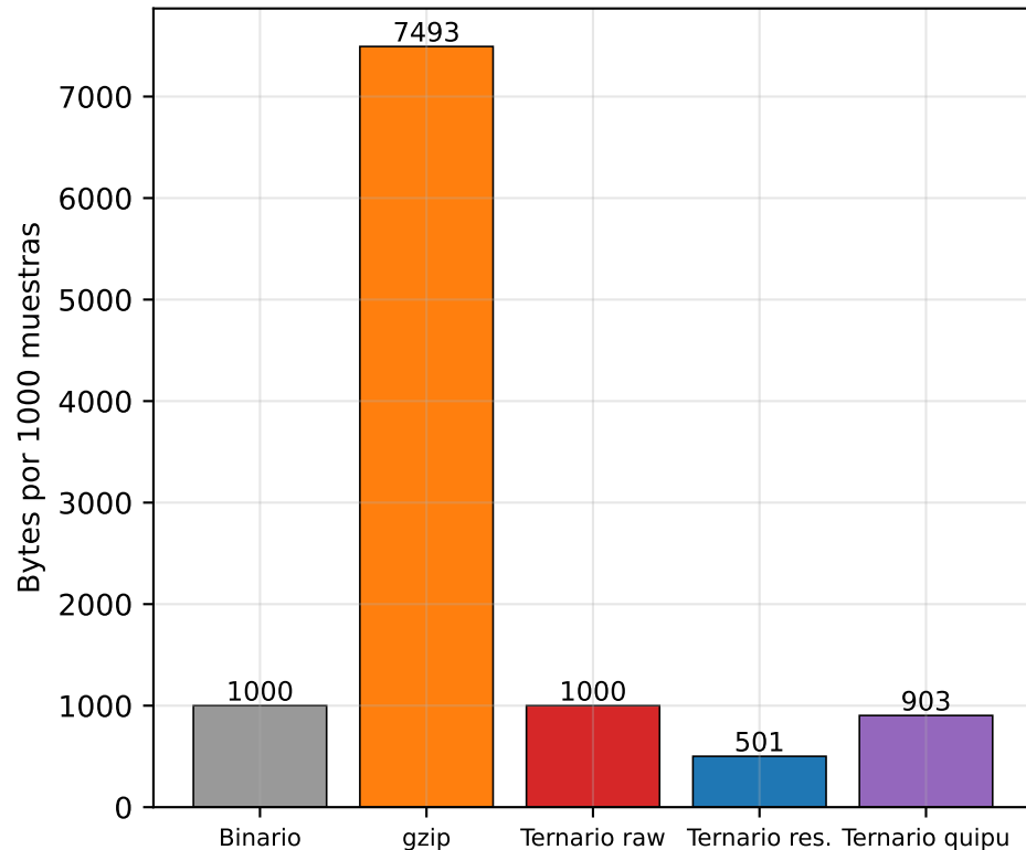
(c) Memoria: ternario residual usa 50% menos
