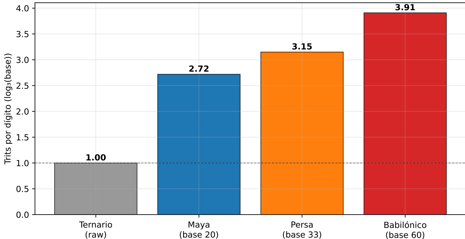
(a) Compresión ancestral: un símbolo babilónico = 3.91 trits (medido)
