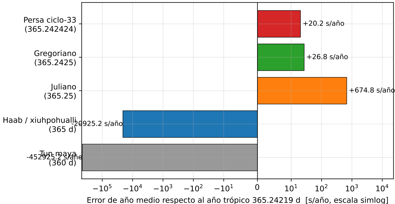
(a) Precisión del año medio: calendarios ancestrales y europeos (cómputo me
