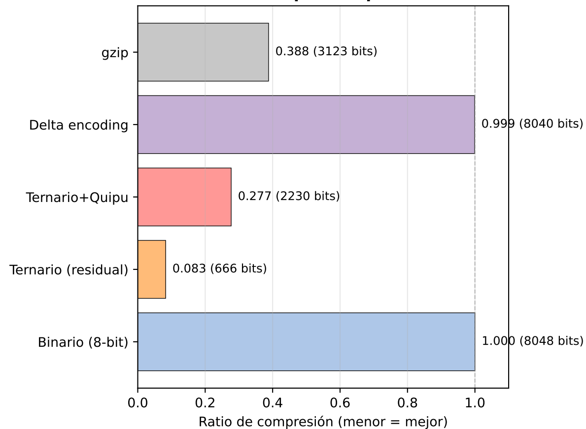
Ratio de compresión por método
