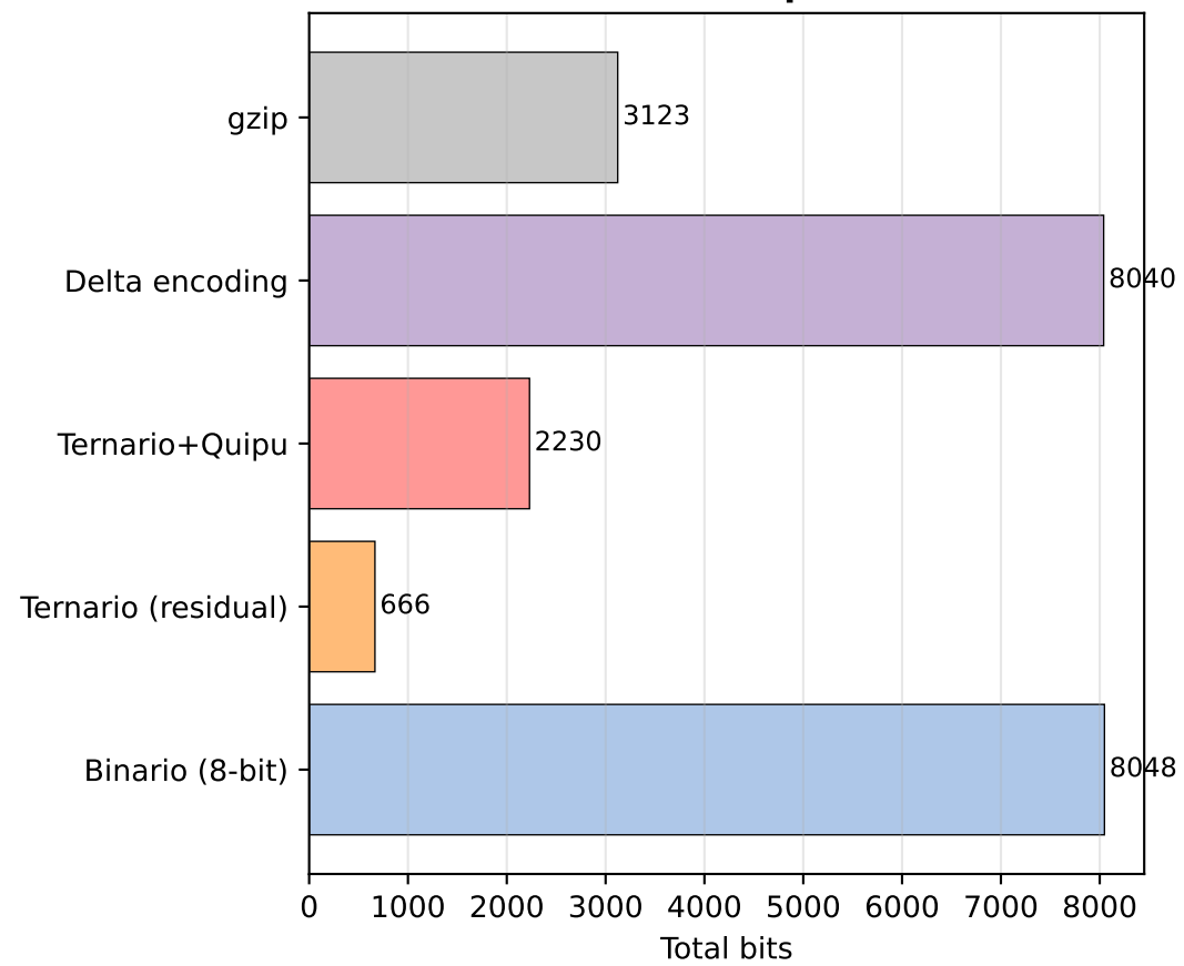
Consumo de bits por método
