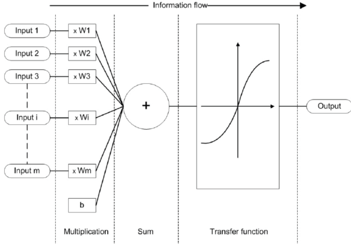
Figura 1.1: Esquema de trabajo de una neurona artificial.
