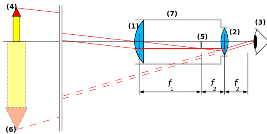
Figura 1.2: Esquema del telescopio Fuente: Michael Schmid. CC BY-SA 2.0 AT
