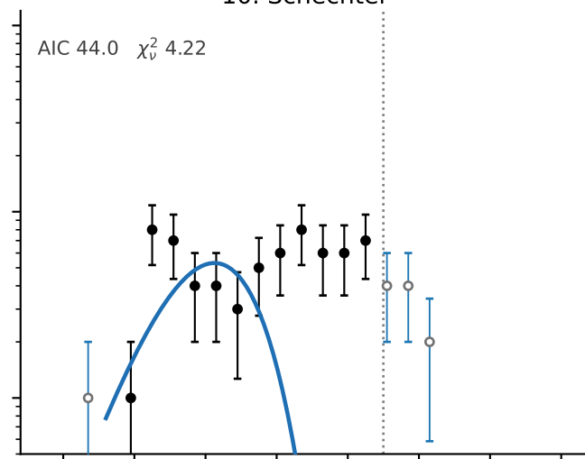
10. Schechter
