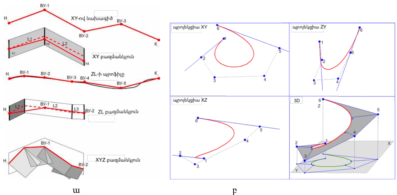
Նկ. 2. Երթուղին, ներկայացված է բազմանկյունների բաժանման տեսքով՝ հատակագծում և պրոֆիլում (ա). ավտոմոբիլային ճանապարհի հենարար կորագիծ մակերևույթի տարրը՝ պրոյեկցիաներում և 3D պատկերում (բ):
