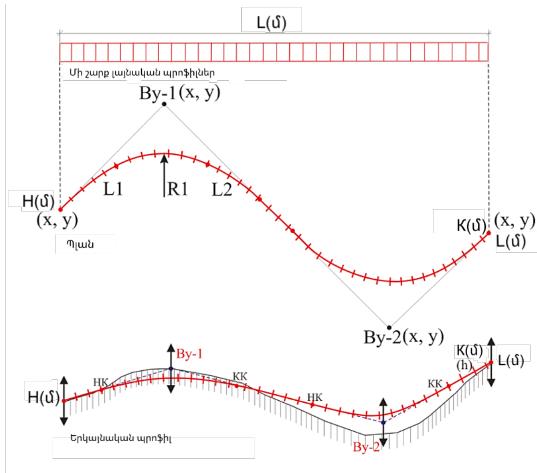
Նկ. 3. Ավտոմոբիլային ճանապարհի երթուղու նախագծային գիծը՝ հաստակագծում (վերևում) և պրոֆիլում (ներքևում)
