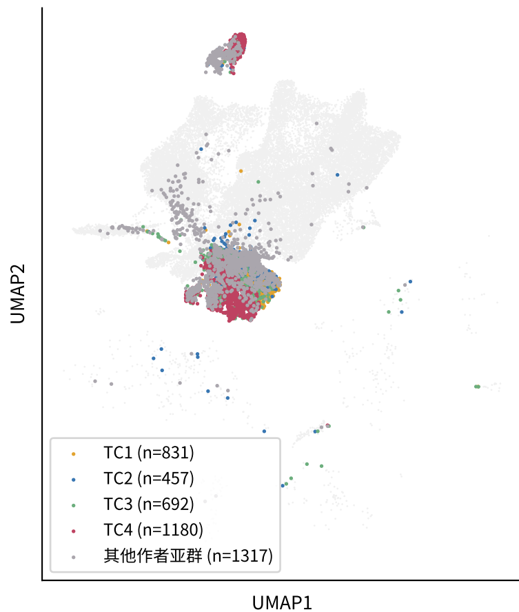
同一批4477个CNA细胞：作者亚群
