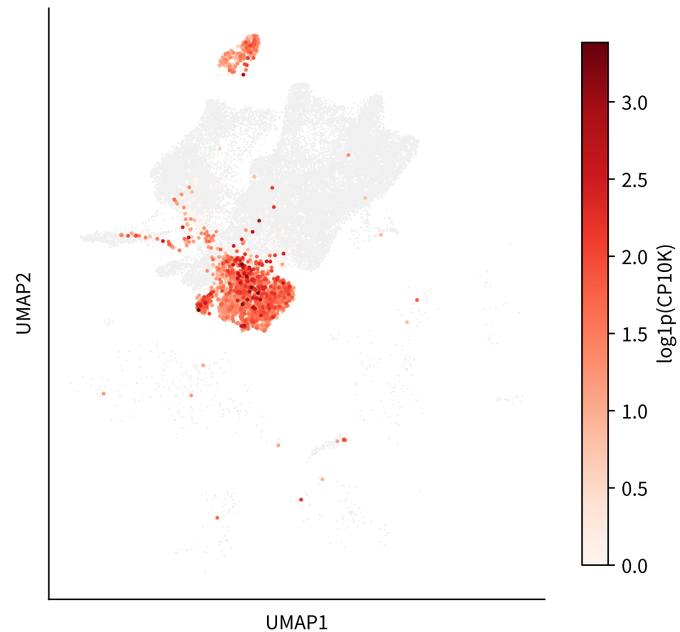
同一坐标：LYPLA1表达
