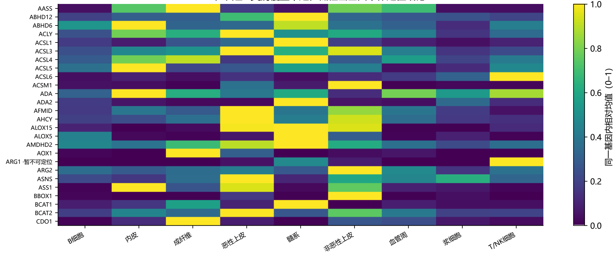
Wu2021; 灰色=类别覆盖不足; 低检出基因不作定位结论
