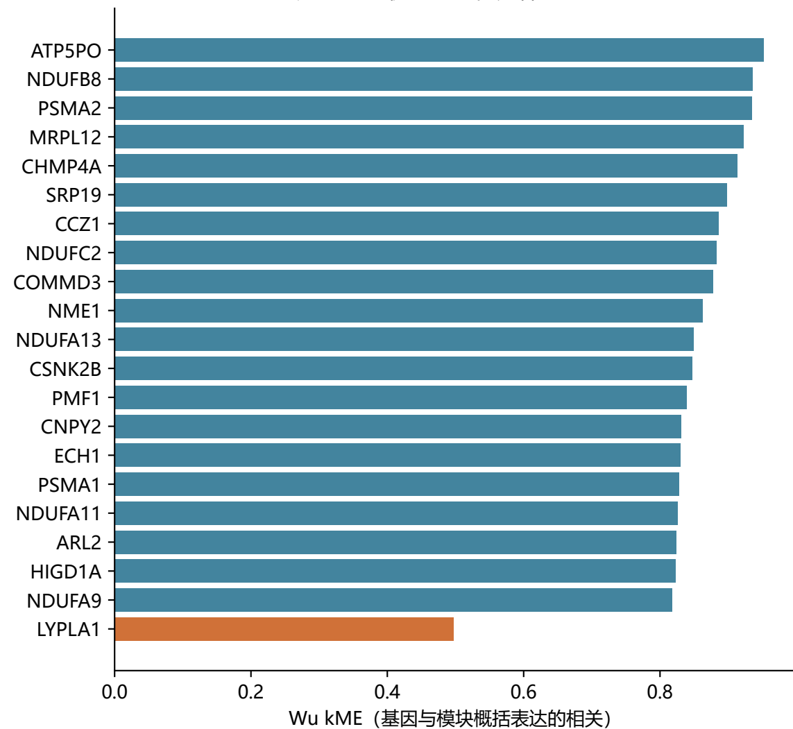
模块内kME最高20个, 另保留LYPLA1
