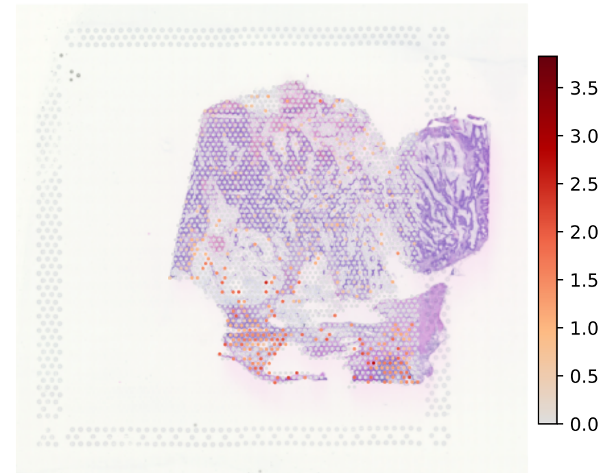
PTPRC | log1p CP10K
