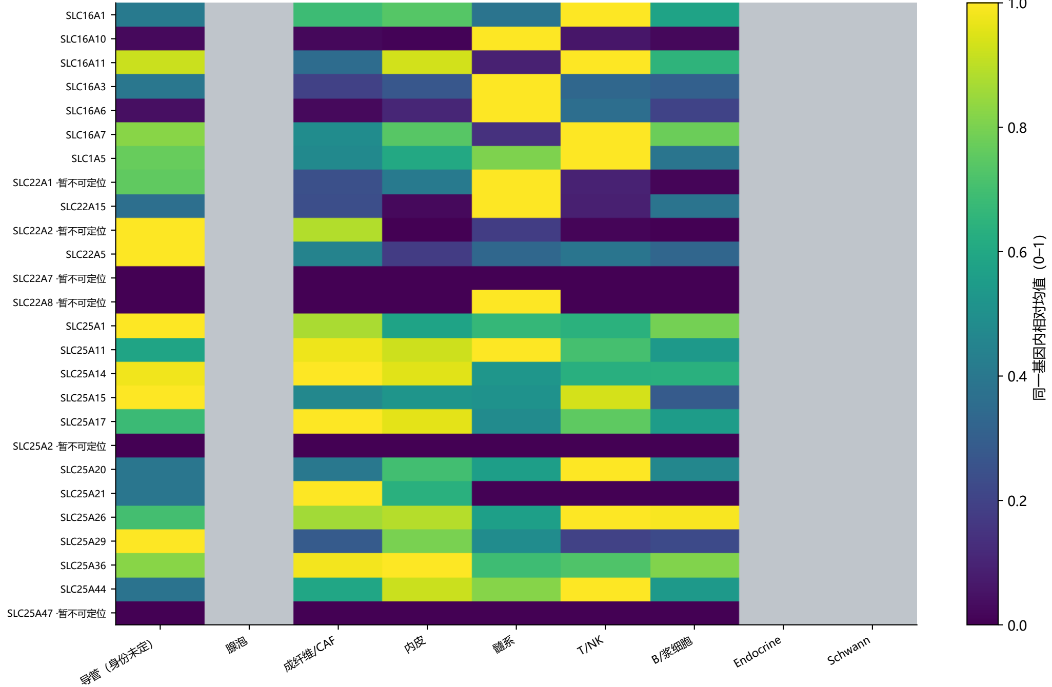
GSE278688; 灰色=类别覆盖不足; 低检出基因不作定位结论
