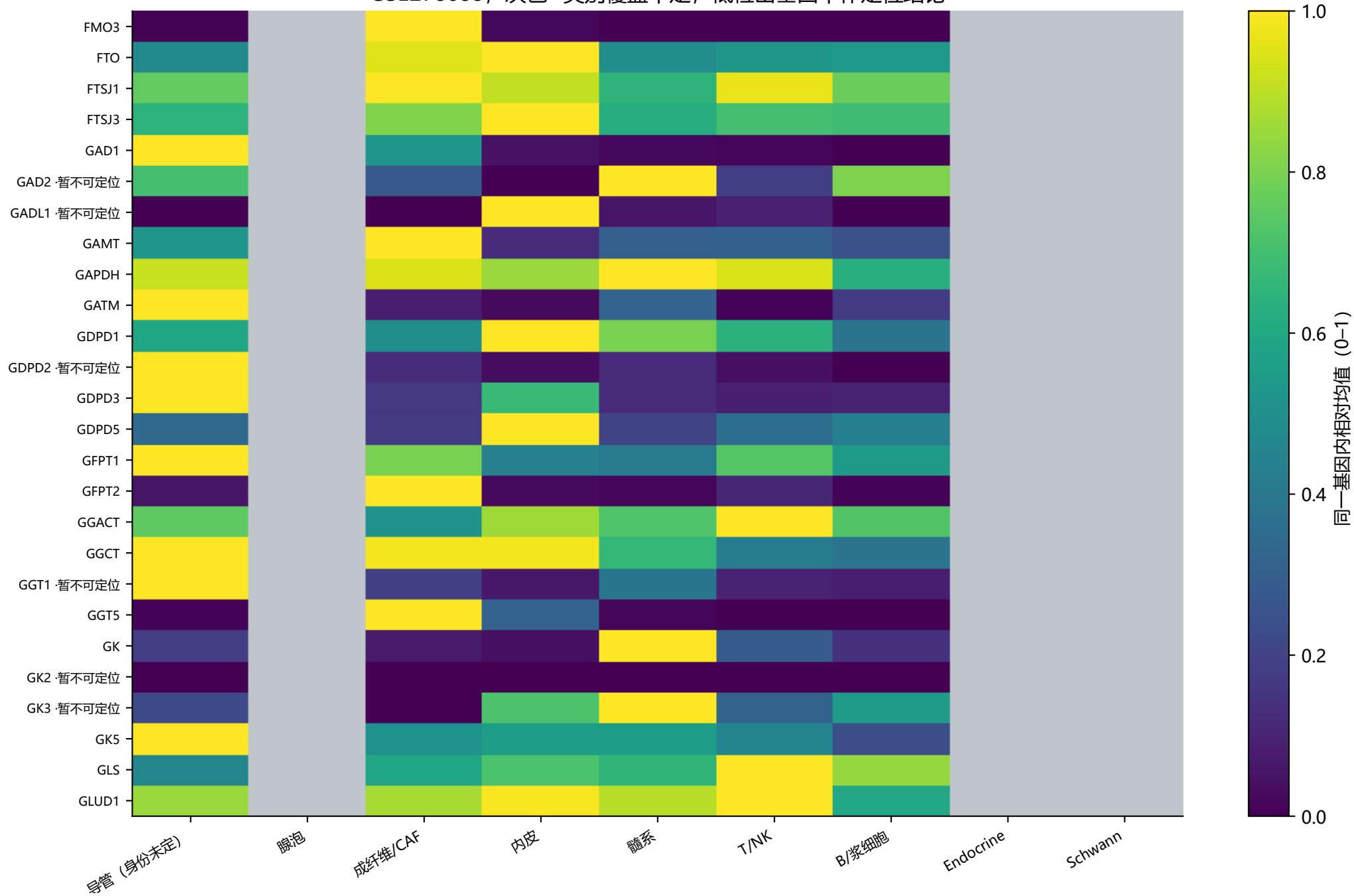
GSE278688; 灰色=类别覆盖不足; 低检出基因不作定位结论
