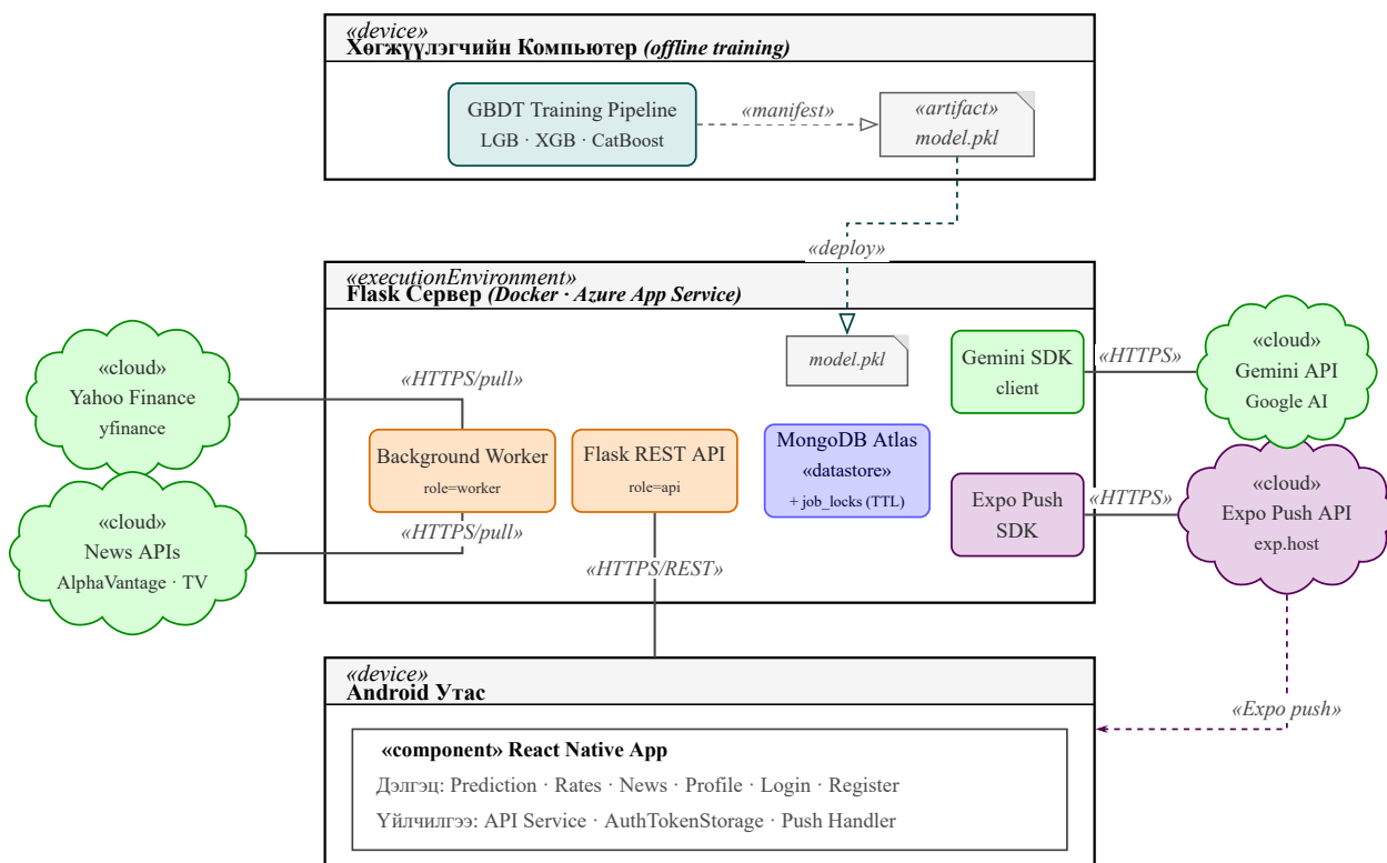
Зураг 3.10 Системийн байршуулалтын диаграмм — Docker, Azure App Service, role-based scaling
