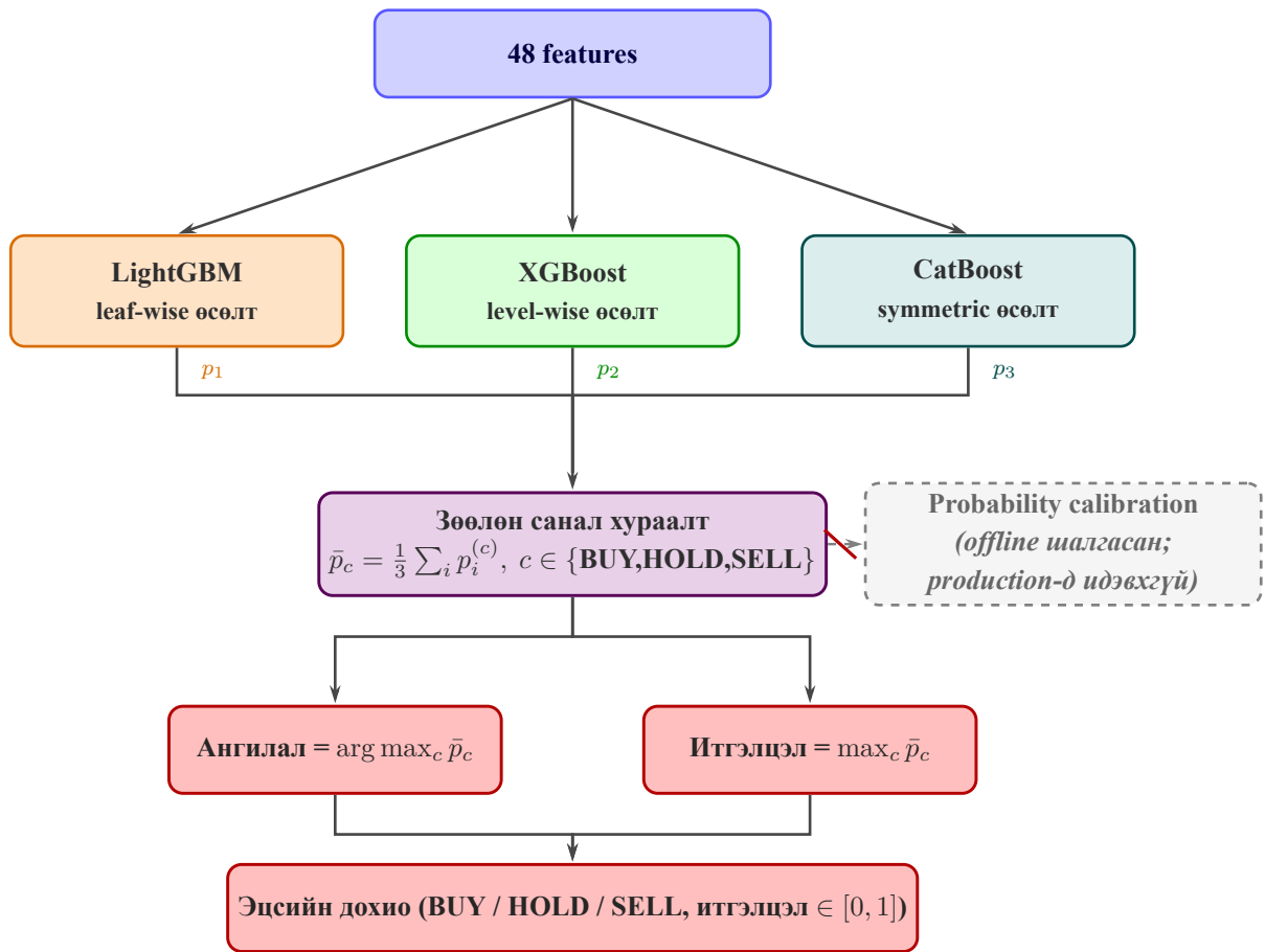
Зураг 3.5 GBDT ансамбль загварын архитектур
