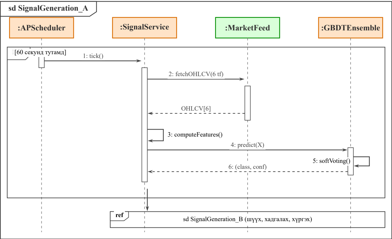
Зураг 3.8 Дохио үүсгэх дараалалтын диаграмм — (А) Таамаглах фаза
