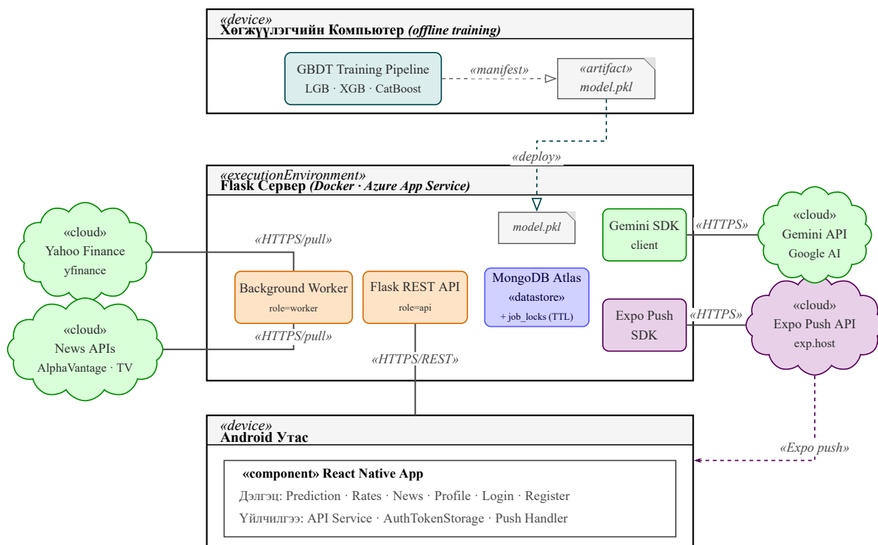
Зураг 3.9 Системийн байршуулалтын диаграмм — Docker, Azure App Service, role-based scaling
