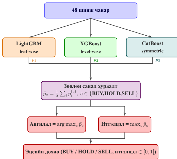
Зураг 2 GBDT ансамбль загварын архитектур
