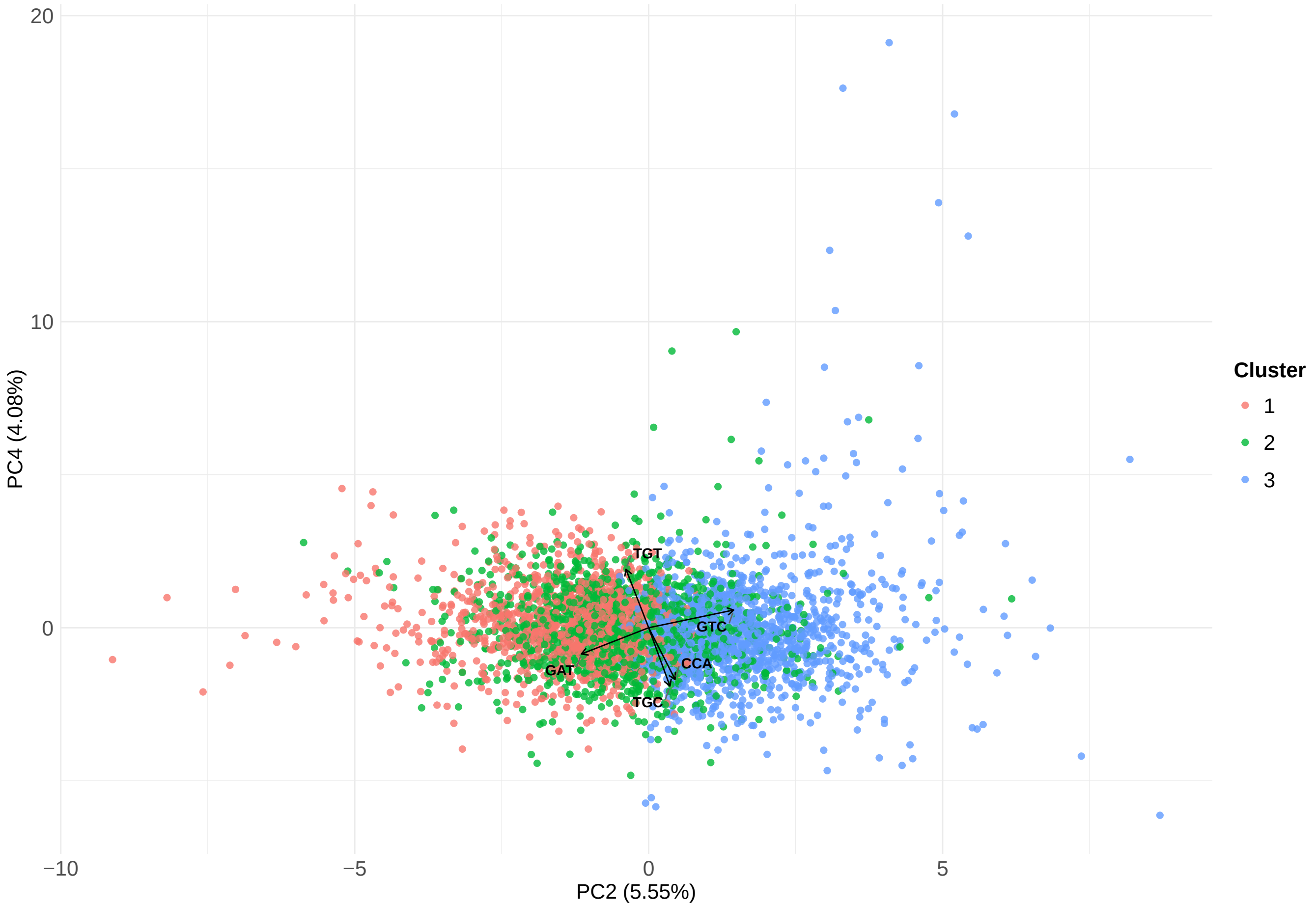
bonobo – genes – PC2 vs PC4
