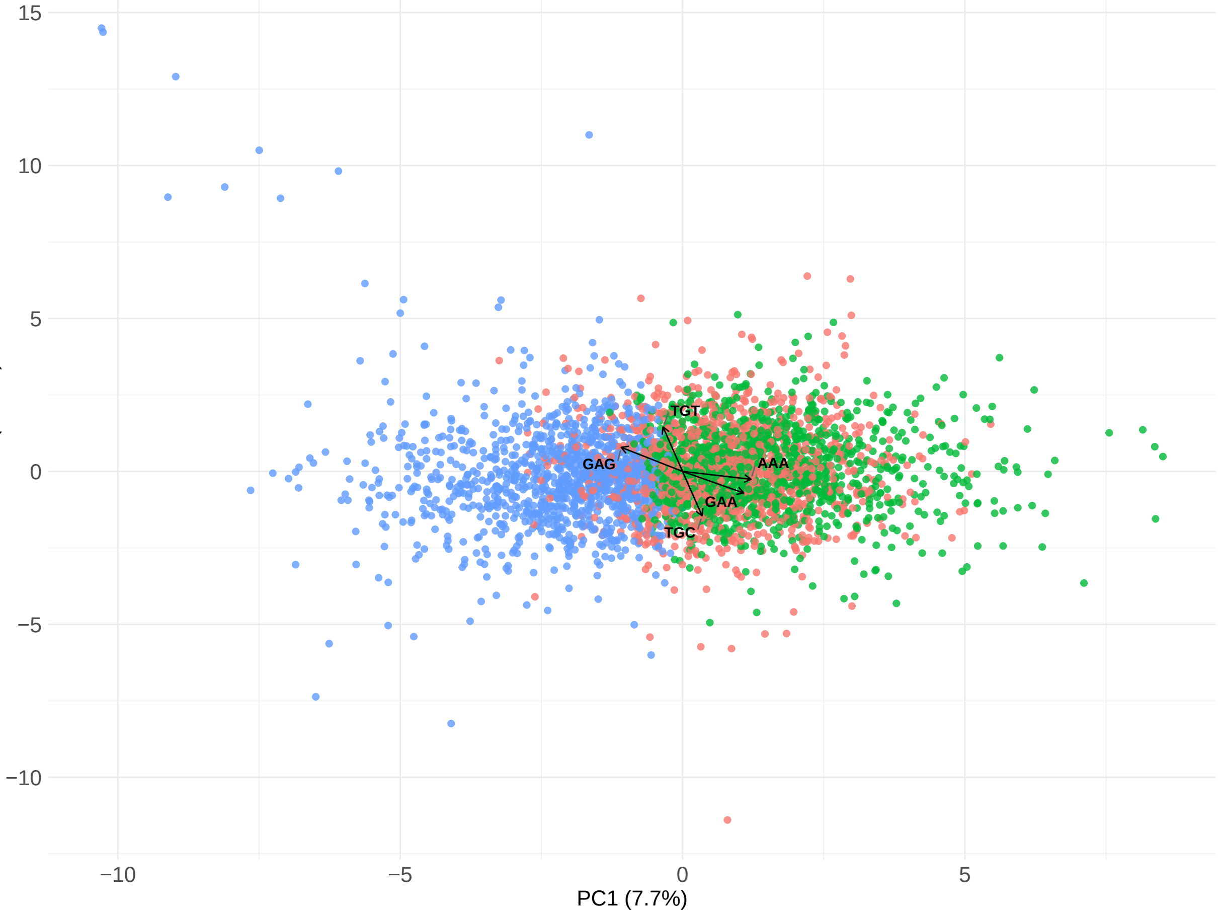
borangutan – genes – PC1 vs PC5
