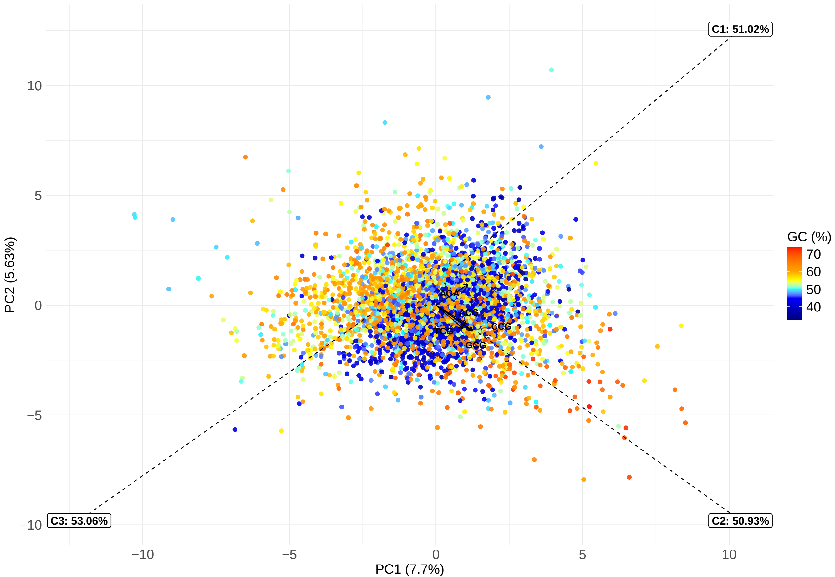
borangutan – genes – PC1 vs PC2
