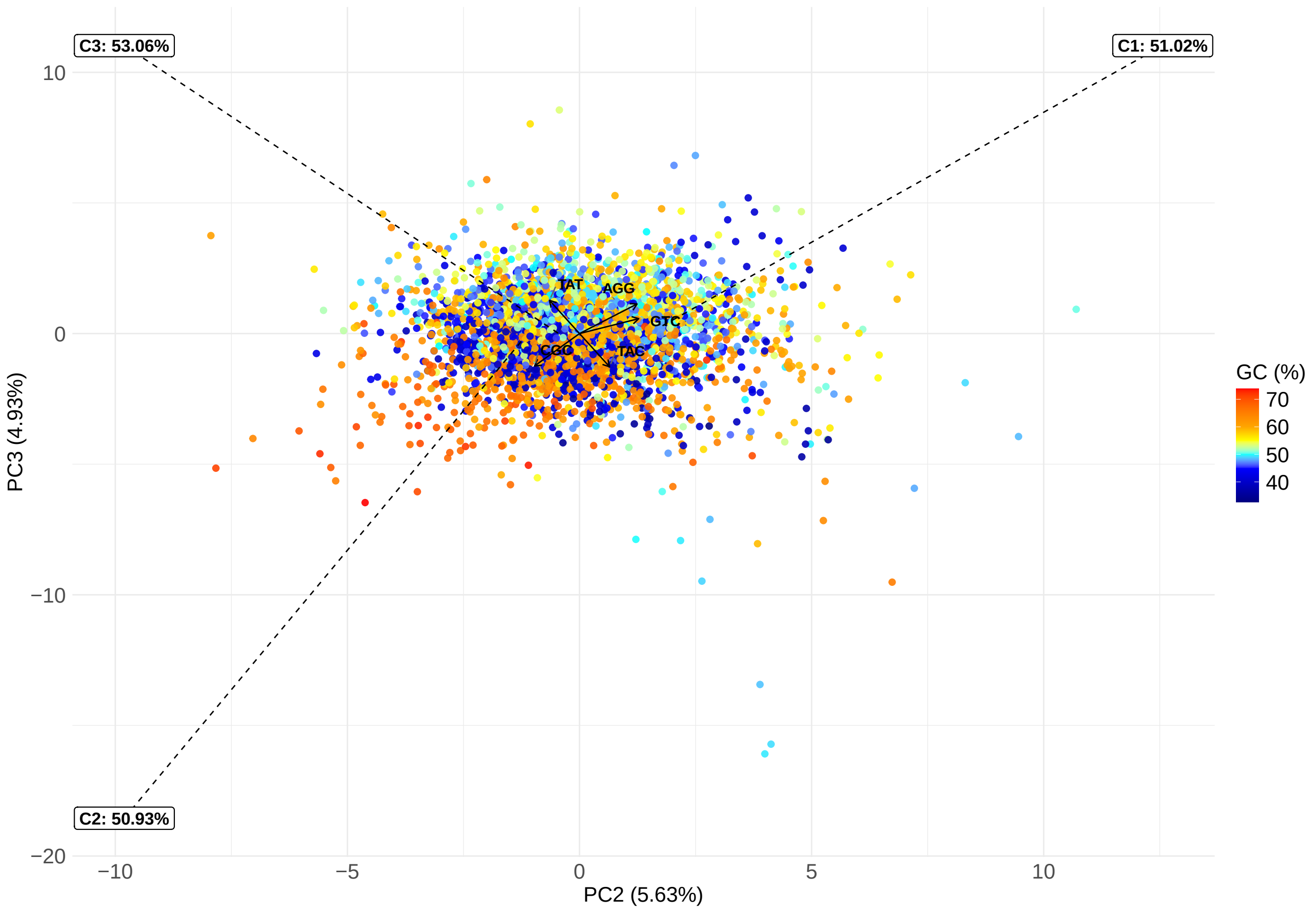
borangutan – genes – PC2 vs PC3
