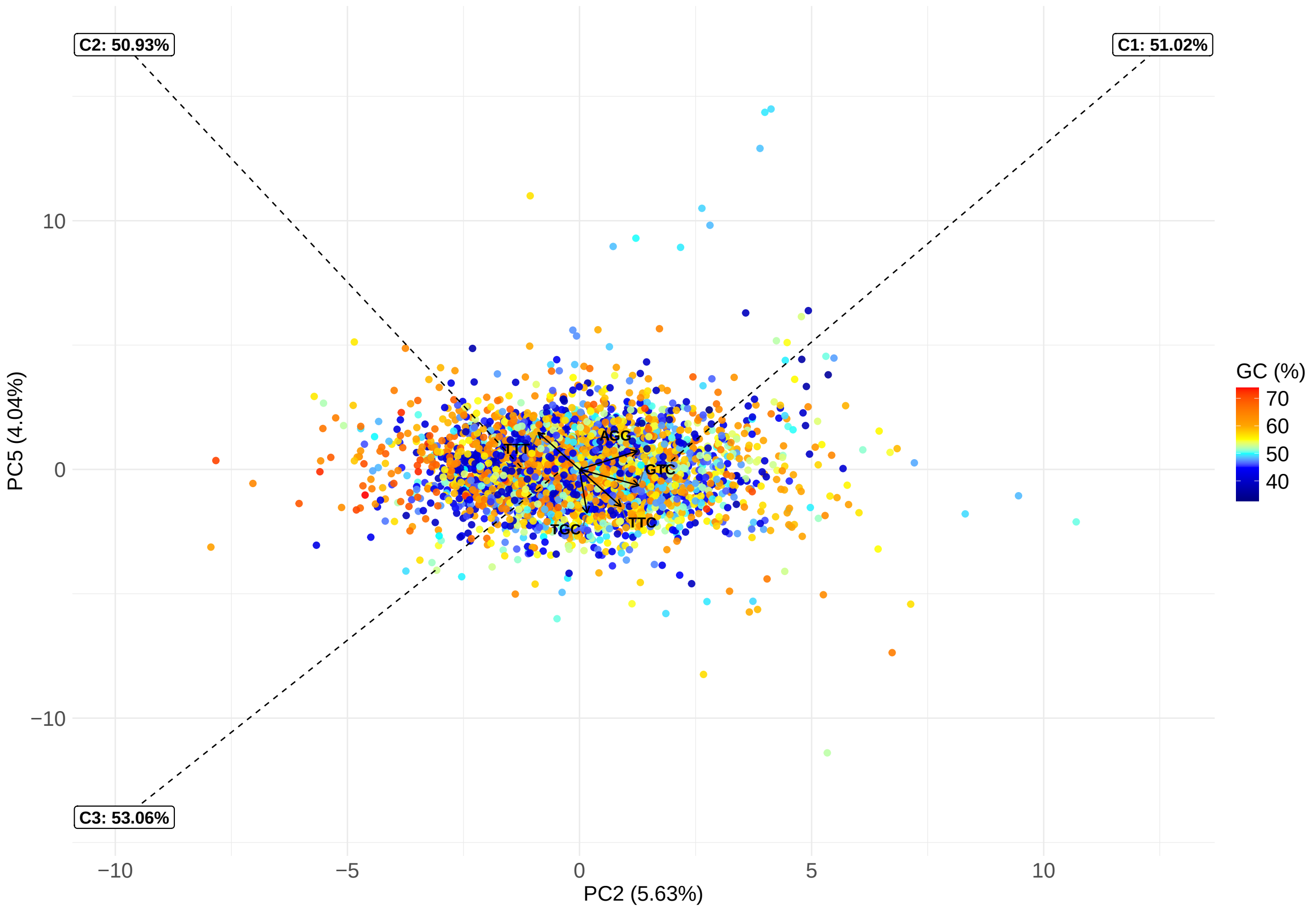
borangutan – genes – PC2 vs PC5
