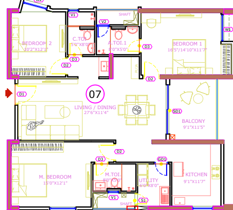
W- TYPE- II 1856 sft
