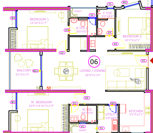
E- TYPE-II 1899 sft
