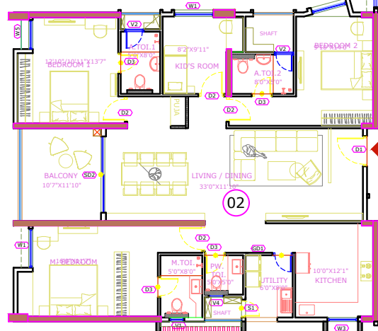
E- TYPE-I 2240 sft
