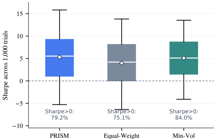
B. Monte Carlo check (e3)
