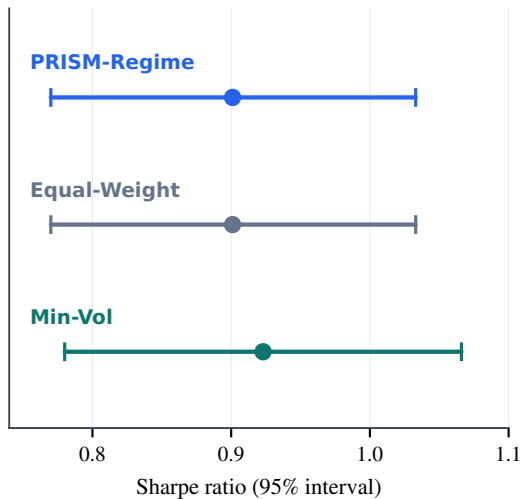
A. Walk-forward check (e3)
