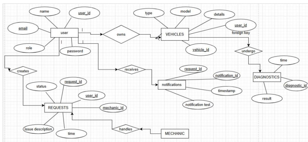
fig13: ER diagram
