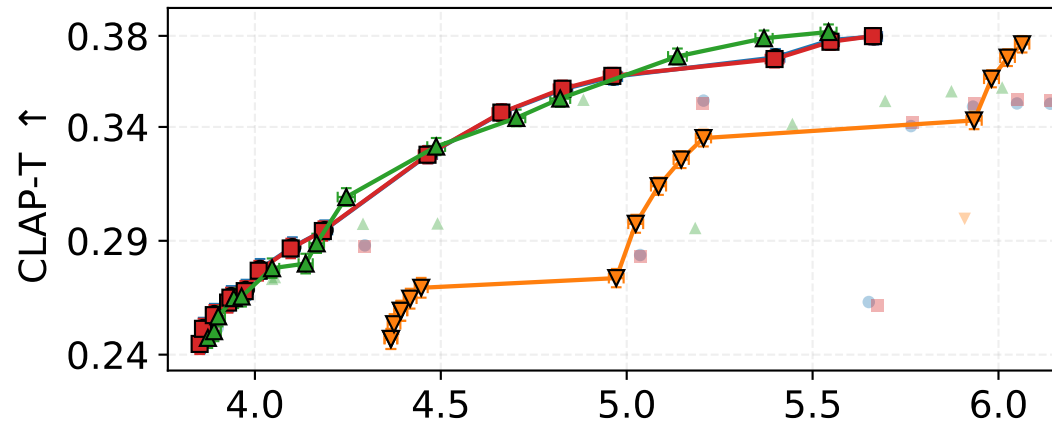
AudioLDM2
