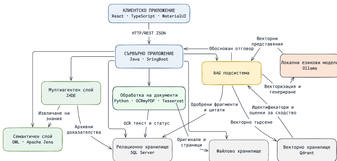
Фигура 4.1. Обща архитектура на системата Ethnowear Източник: авторска разработка.
