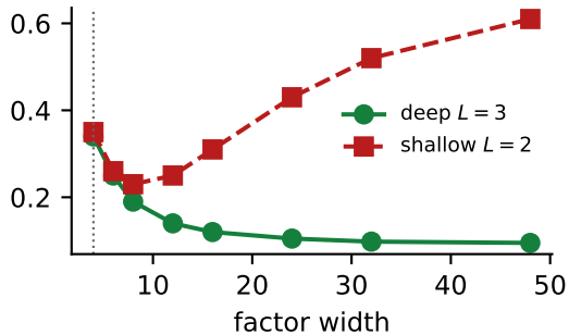
Test error
