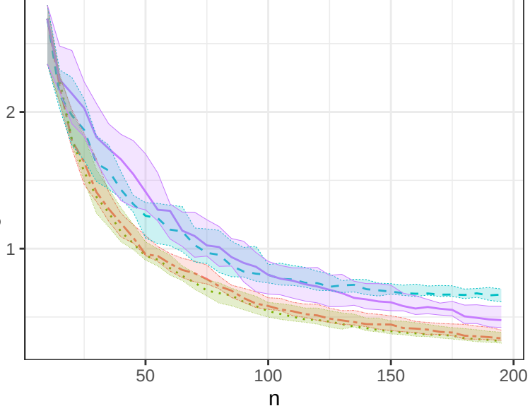
Kullback–Leibler(SLGP, Bin)
