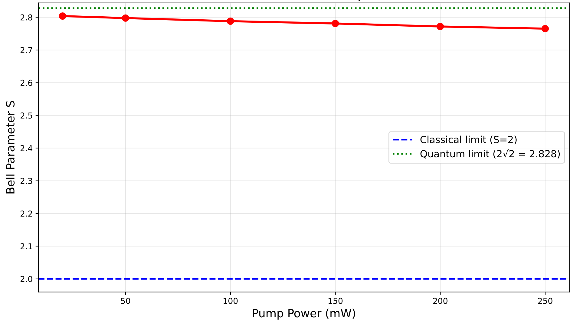
Bell Parameter S vs Pump Power
