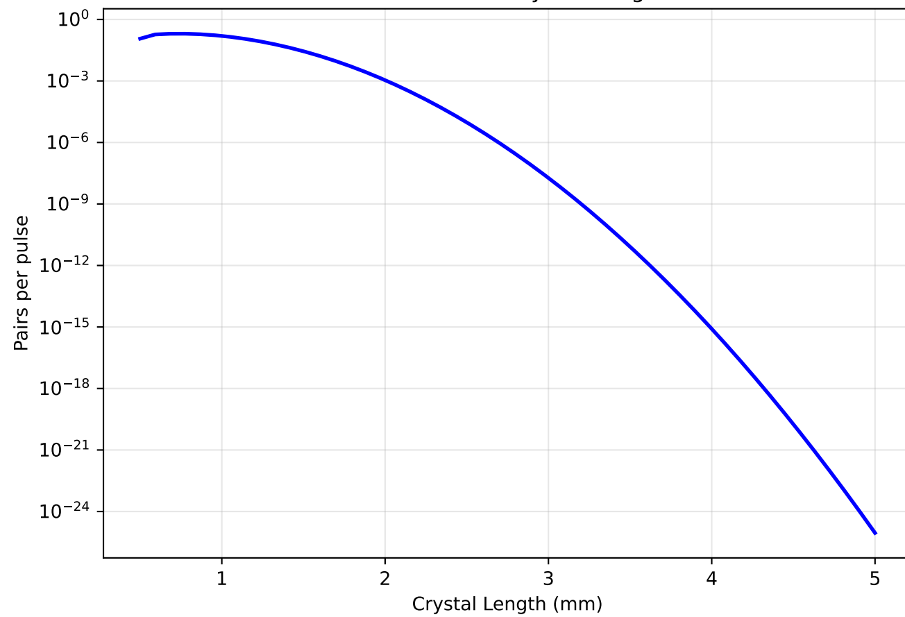
SPDC Pairs vs Crystal Length
