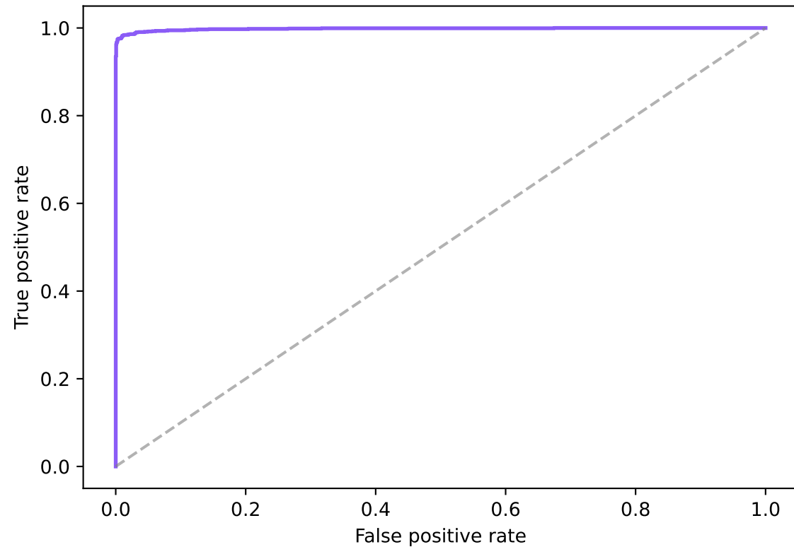
ROC (AUC=0.9981)
