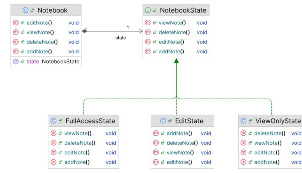
Рис. 2 — Діаграма класів
