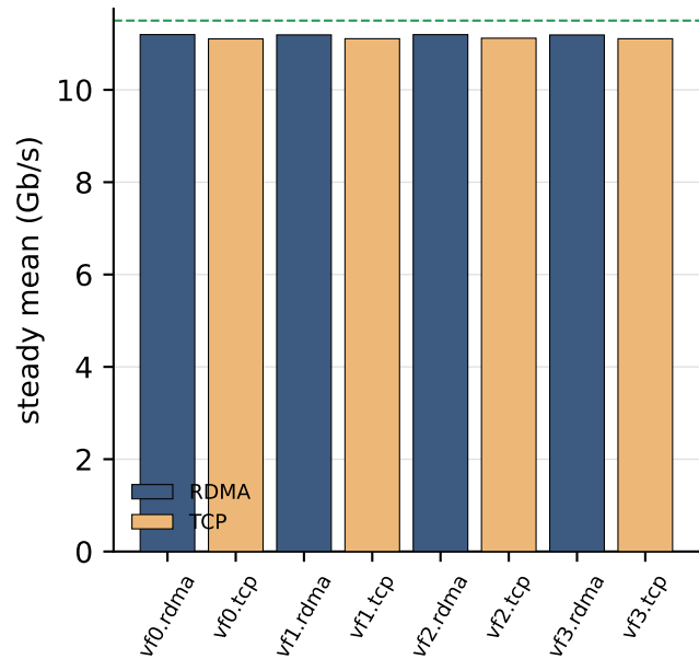
Jain=1.000 agg=89G
