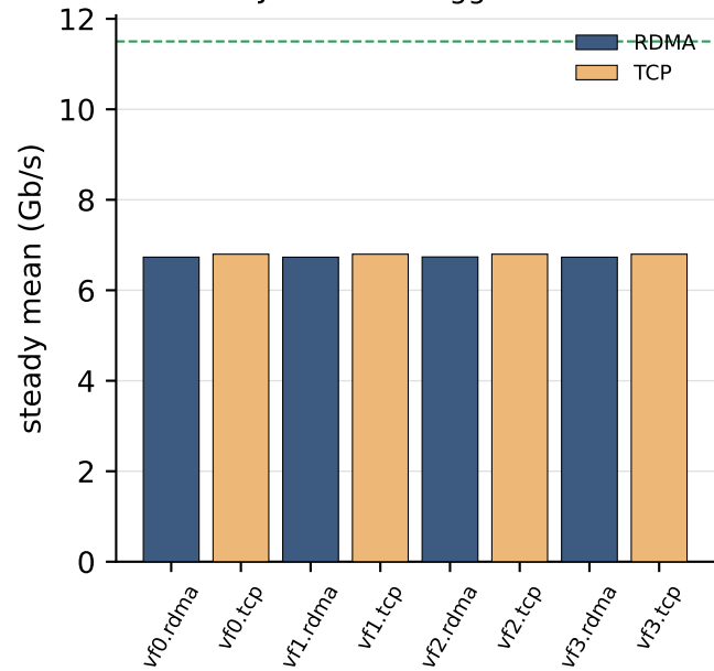
Jain=1.000 agg=54G
