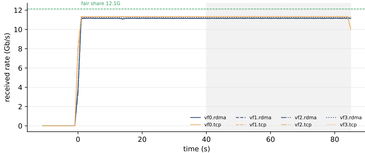
incast8 — RDMA SEND/RECV
