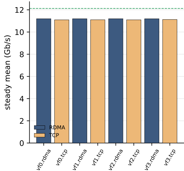
Jain=1.000 agg=89G
