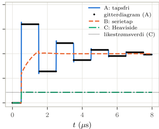
(b) Åpen ende, R_s = Z_0/4
