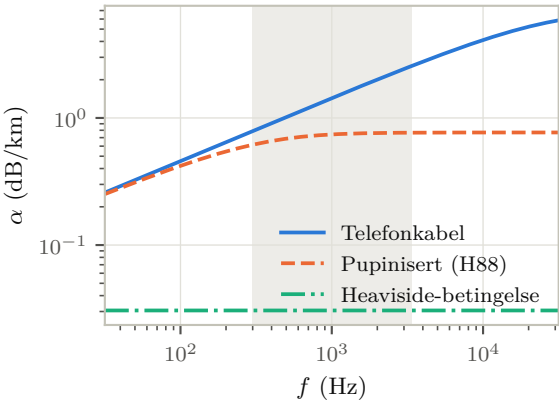
(a) Dempning
