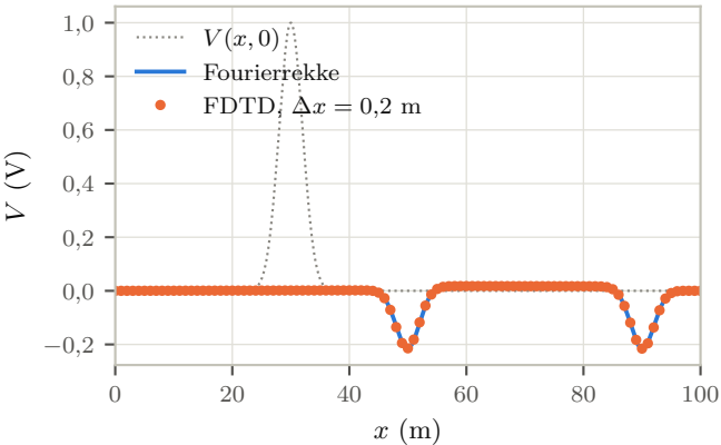
(a) Tilfelle B, t = 0,4 \mu\text{s} , kortsluttede ender
