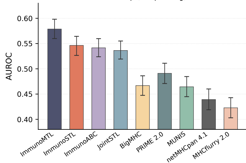
Bootstrap (1:5 pos:neg)
