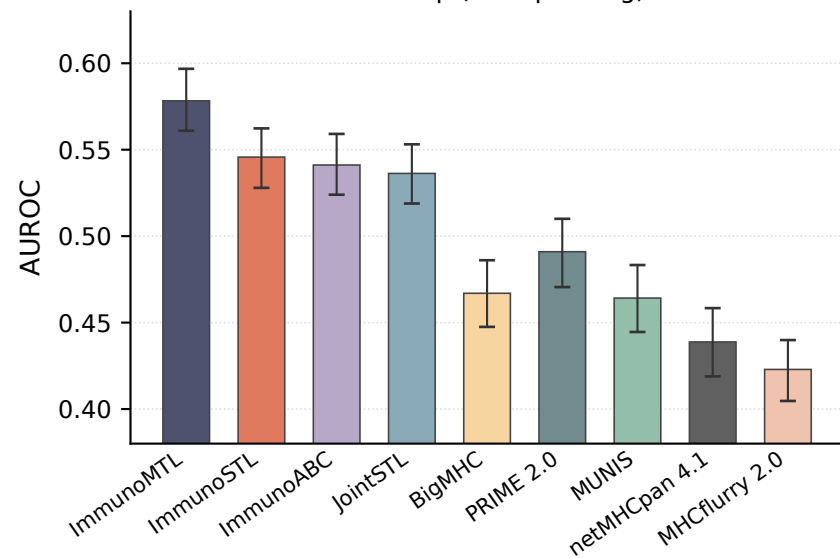
Bootstrap (1:10 pos:neg)
