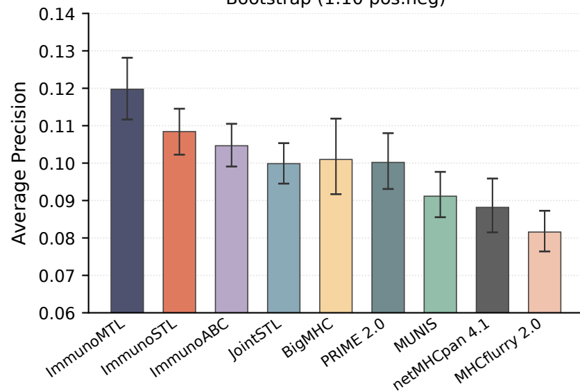
Bootstrap (1:10 pos:neg)
